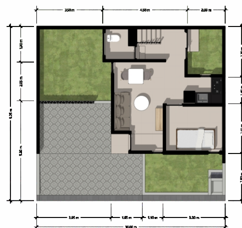
Lantai 2
